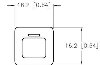
GASKET
